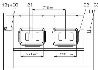
RÜCKANSICHT MB 66
