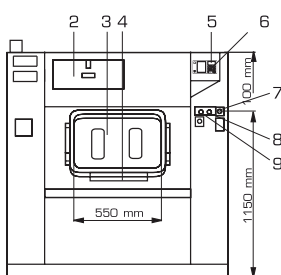
FRONTANSICHT MB 16 26 33 44
