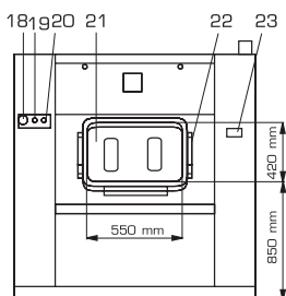
RÜCKANSICHT MB 16 26 33 44
