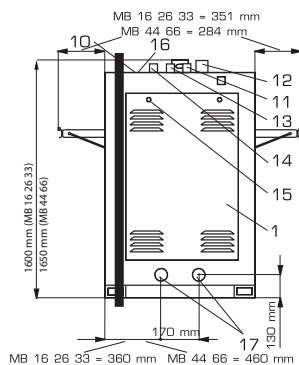
RÜCKANSICHT MB 66
