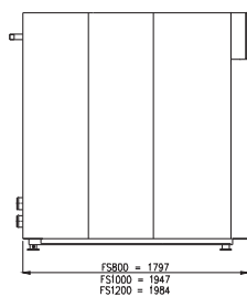
SEITENANSICHT FS800 1000 1200
